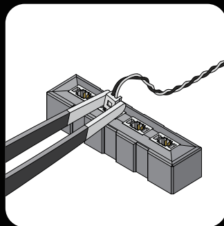
3. 轻轻地左右晃动连接器。
