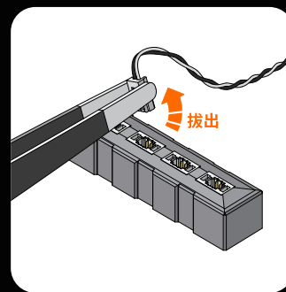
5. 拔下连接器。
